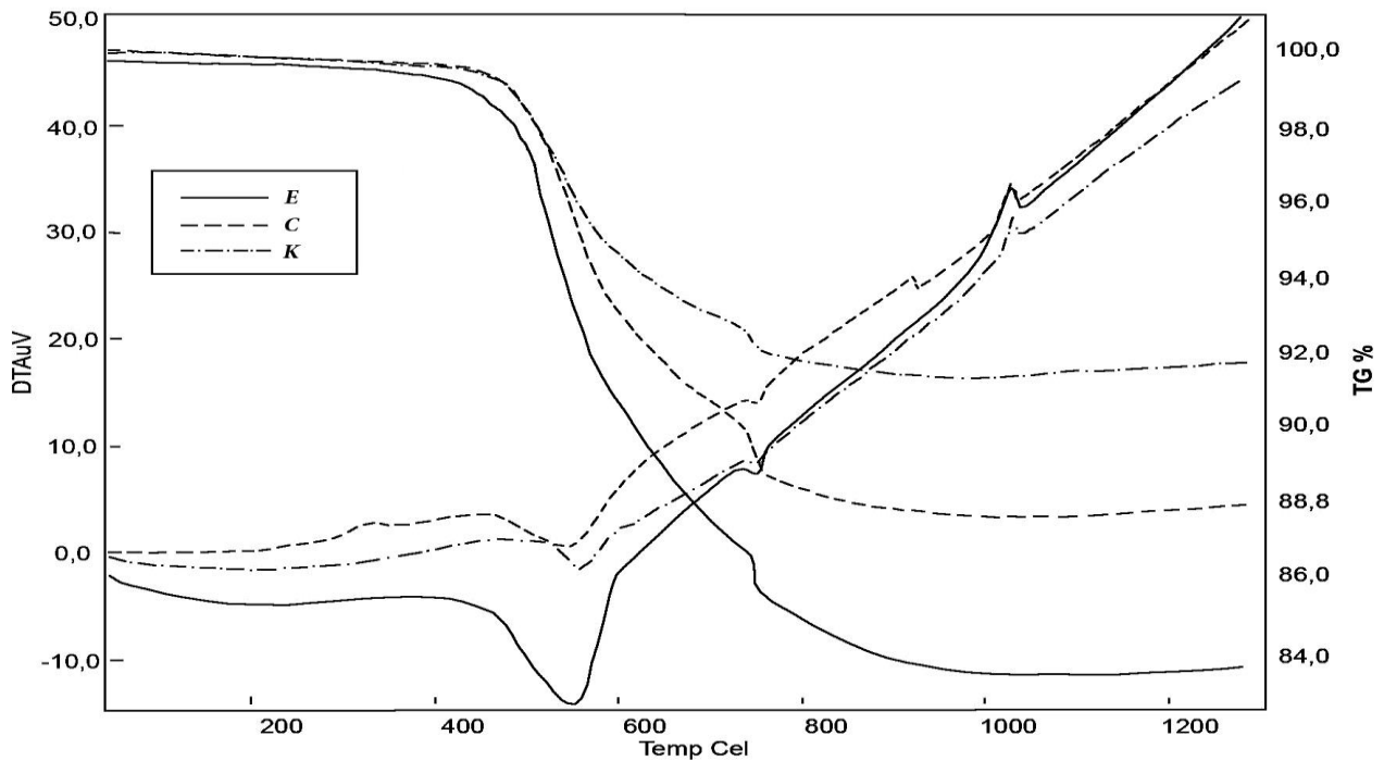
Şekil 2. K, E ve C kaolinlerinin TG-DTA eğrileri.
