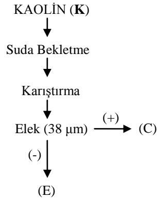
Şekil 1. E ve C kaolinlerinin üretim işlemleri.
