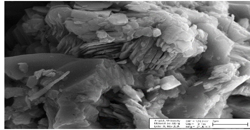
Şekil 4. E kaolininin SEM görüntüsü.
