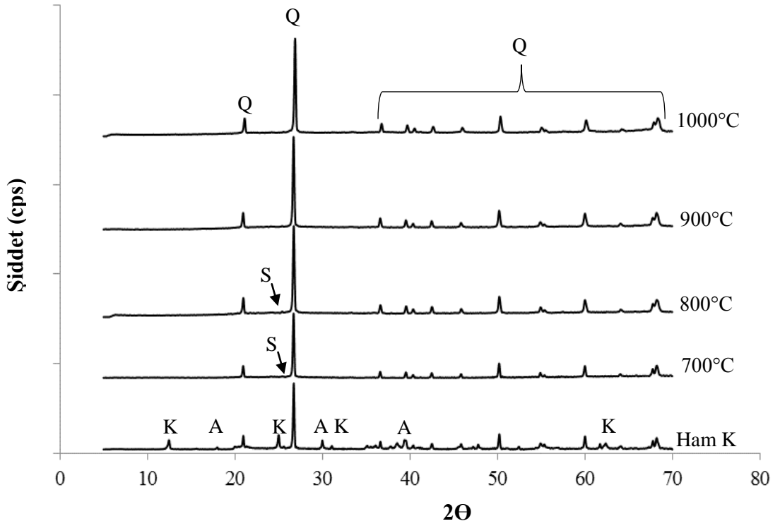
Şekil 7. Ham ve kalsine K kaolinlerinin XRD paternleri (K: kaolinit, A: alunite, Q: kuvars, S: KAl(SO_4)_2 ).
