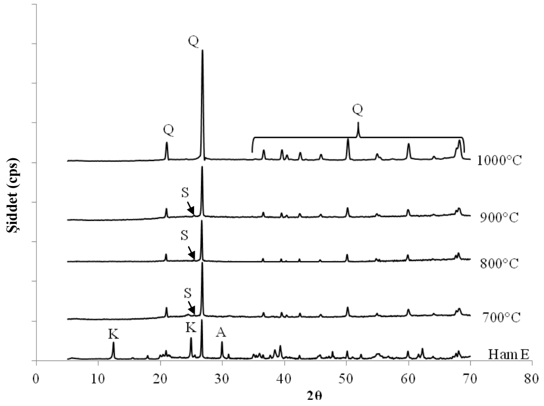
Şekil 8. Ham ve kalsine E kaolinlerinin XRD paternleri (K: kaolinit, A: alunite, Q: kuvars, S: KAl(SO_4)_2 ).
