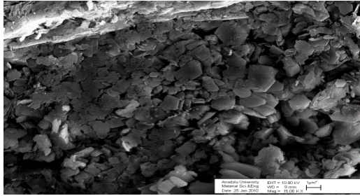
Şekil 3. K kaolininin SEM görüntüsü.
