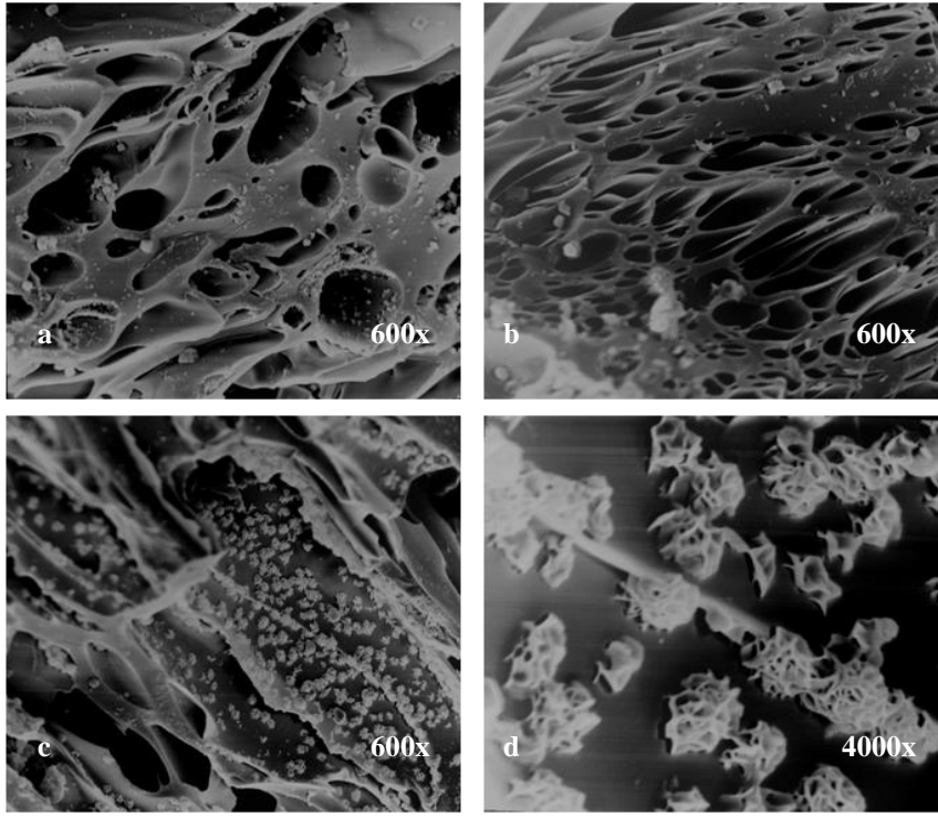
Şekil 1. Bir pomza* örneğinin taramalı elektron mikroskop görüntüsü [11]. *Pomza örneği İzmir-Menderes yöresine aittir.
