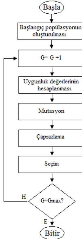
Şekil 1. FGA akış şeması
