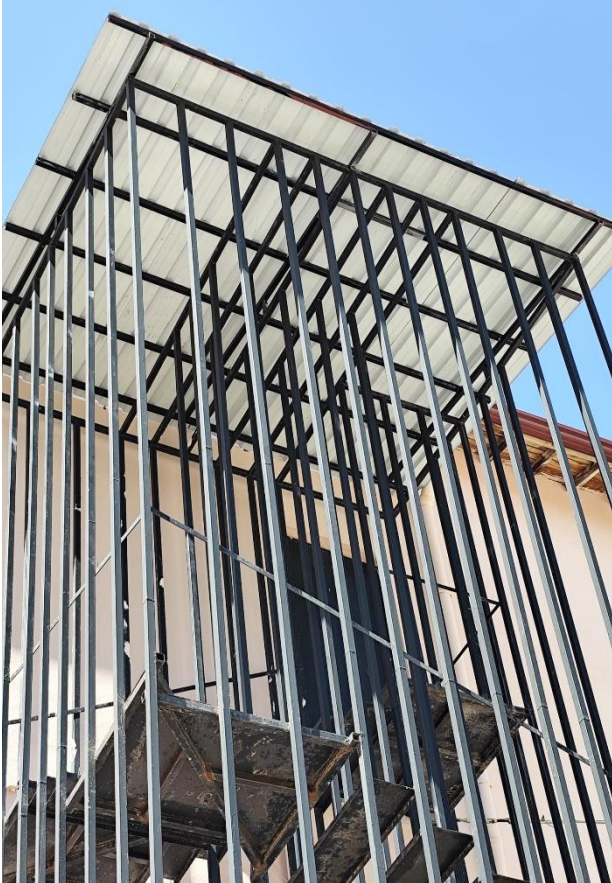
Pazarlar MYO. Yangın Merdiveni Trapez Saç Çatı Örtüsü İmalatı
